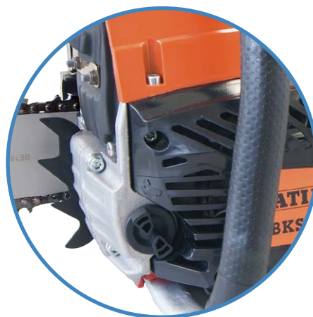
Carter de réservoir d'huile renforcé Griffes de maintien acier trempé
