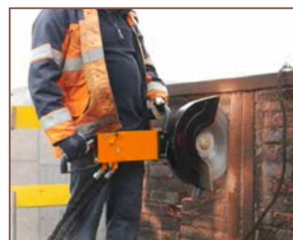
Coupe verticale et horizontale
