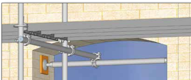
Amarrage en fenêtre avec : lot étrésillon + colliers à clavettes ou raccords à boulons + tubes + cales bois.
