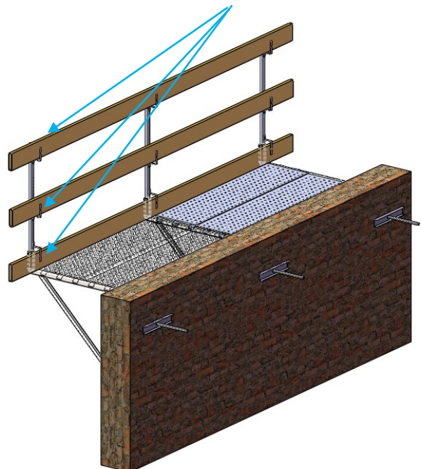
Installation des planches en bois (garde-corps principale, intermédiaire, plinthe); puis, fixation avec des clous ou des vis
