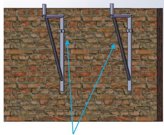
Installation des consoles de façade avec espacement maximale 160 cm
